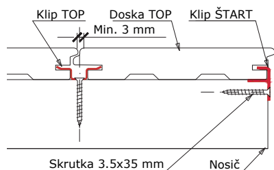
Obr. 3 Kotvenie terasových dosiek TOP pomocou nerezových klipov a skrutiek
